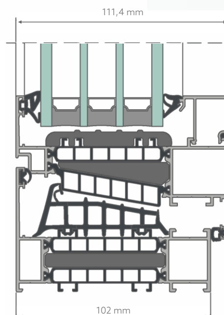
PRZEKRÓJ PRZEZ OKNO TM 102HI
